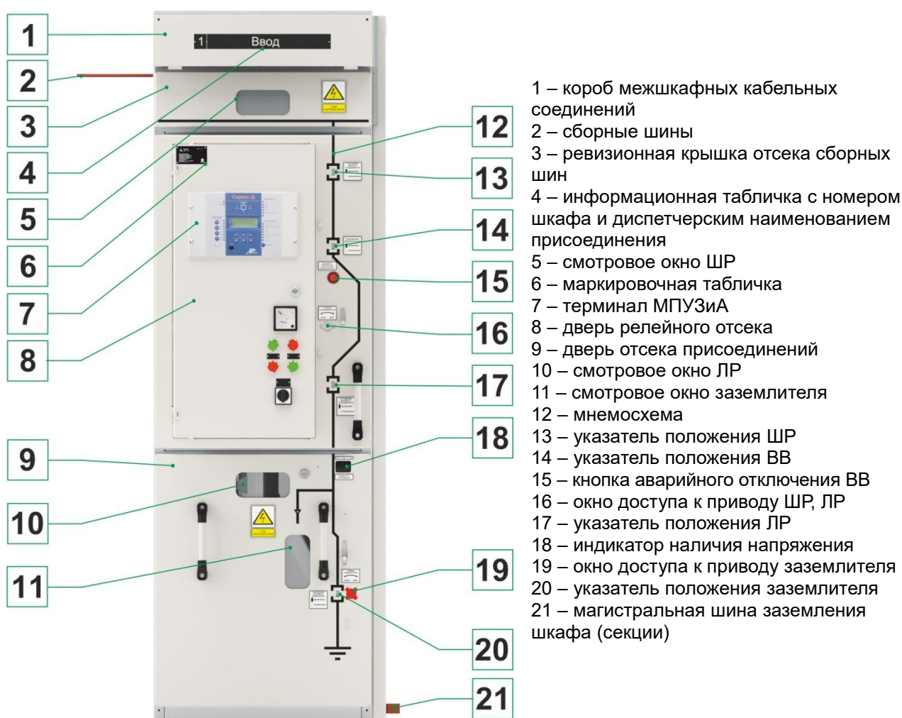
Рис. 1.1 Вид шкафа КСО с фасада
