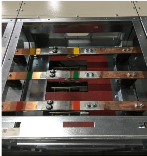
Рис. 2.2 Последовательность монтажа сборных шин секции
