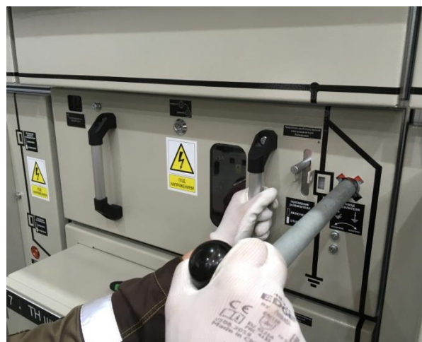
Рис. 2.13 Размещение рычага переключения заземлителя
