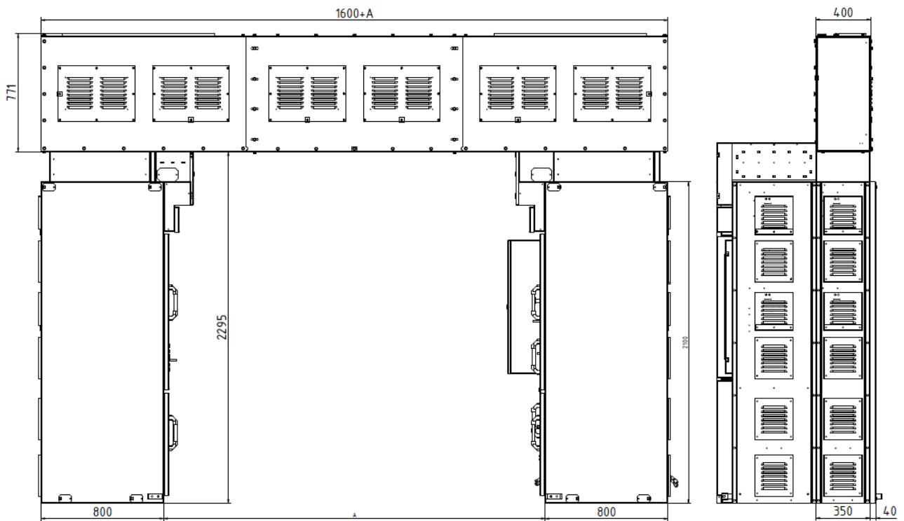
Рис. П5.7 Шинный мост с боковых приставок
