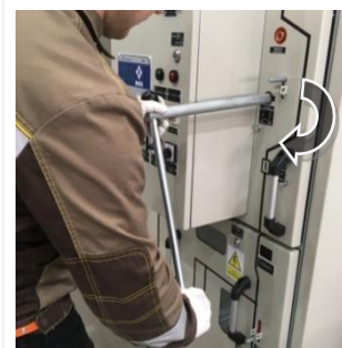
Рис. 2.34 Поворот рычага переключения
